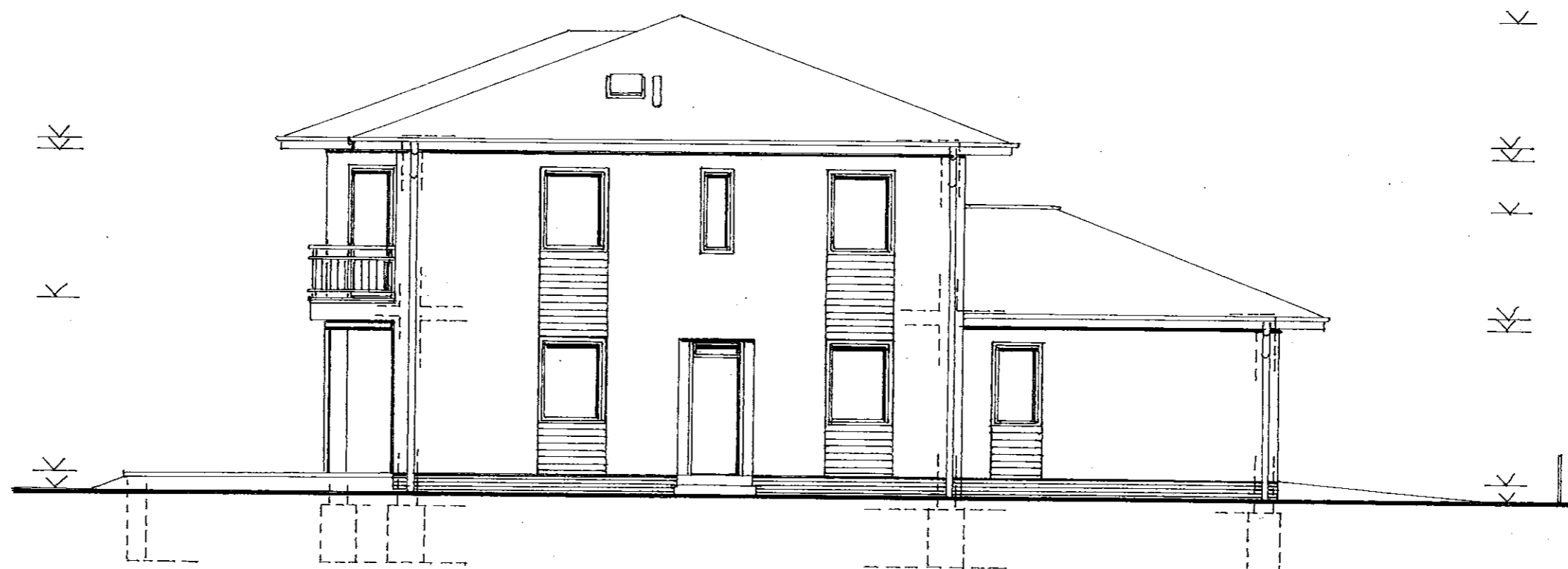
északkeleti homlokzat 1:100
